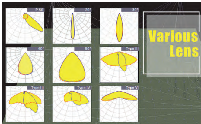
Optionale Linsen mit verschiedenen Abstrahlwinkeln Optional lenses with different beamangles Lentilles en option avec différents angles de faisceau Optionele lenzen met verschillende stralingshoeken
