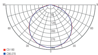
light distribution curve nach oben
