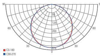
light distribution curve nach oben
