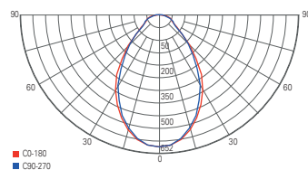
light distribution curve nach unten
