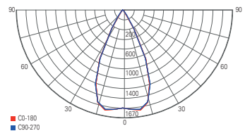
light distribution curve nach unten
